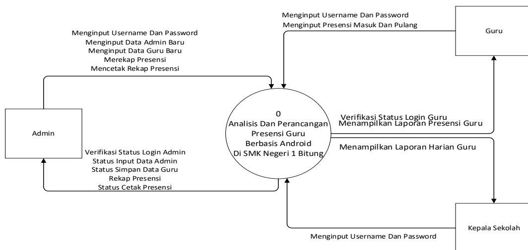
Gambar 1. Diagram Konteks
