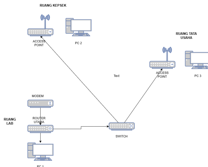
Gambar 2. Topologi Jaringan SMK Kristen Getsemani Manado
