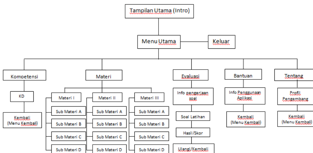
Gambar 2. Struktur Hirarki Menu Aplikasi Pembelajaran
