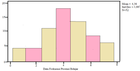
Gambar 2.3 Histogram Prestasi Belajar Siswa
