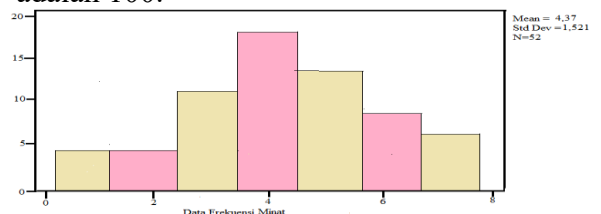
Gambar 2.2 Histogram Minat Belajar
