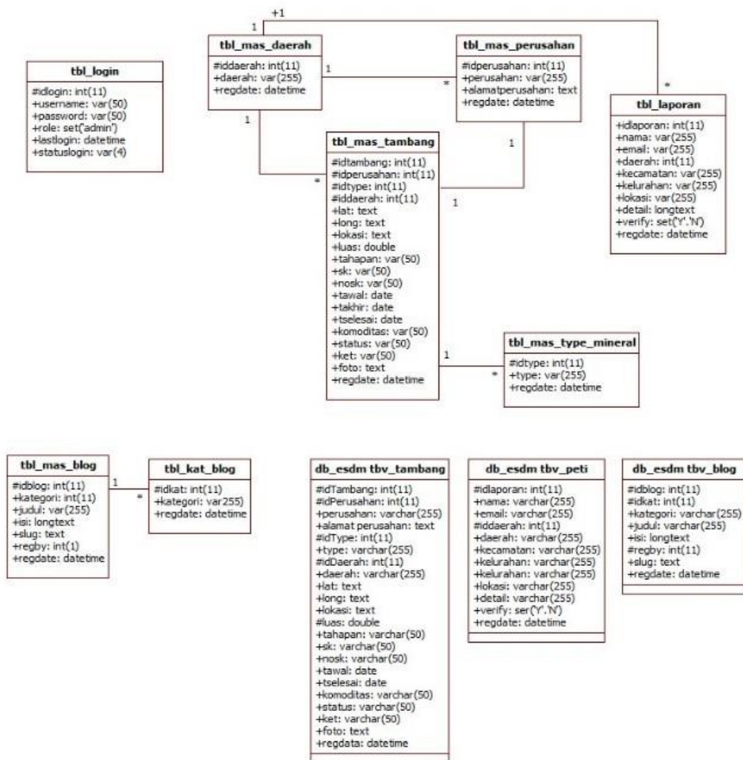
Gambar 5. Class Diagram Pemetaan Pertambangan
