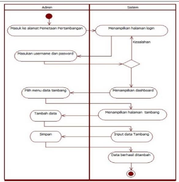
(b) Activity Diagram Tambah Data Pertambangan
